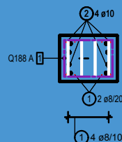
Schnitt A - A
