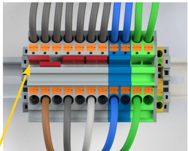
Abbildung 3: einfache Zuleitung
