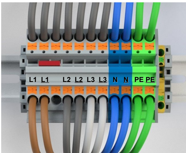
Abbildung 2: zweifache Zuleitung
