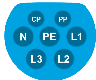
Abbildung 4: Typ 2 Stecker weiblich
