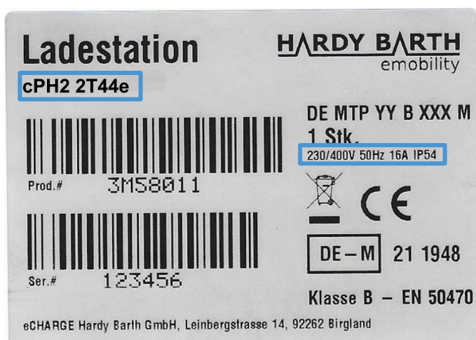
Abbildung 1: Typenschild cPH2
