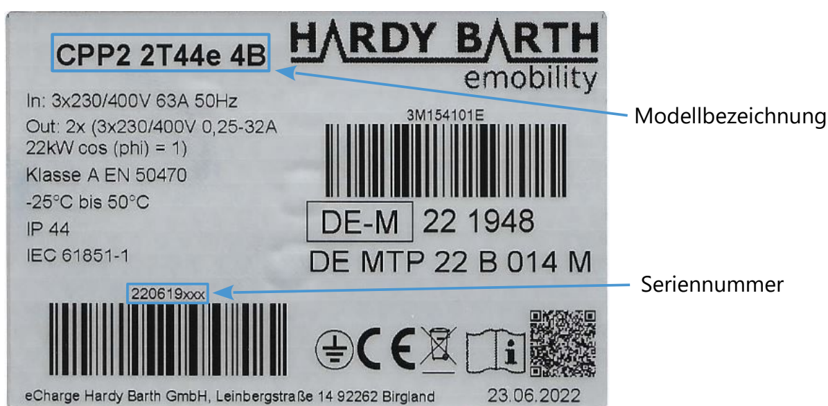
Abbildung 1: Typenschild cPP1*
