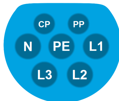
Abbildung 2: TYP 2 Stecker Weiblich
