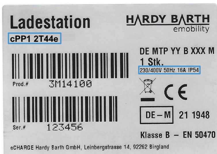
Abbildung 1: Typenschild cPP1
