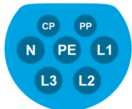
Abbildung 2: TYP 2 Stecker Weiblich
