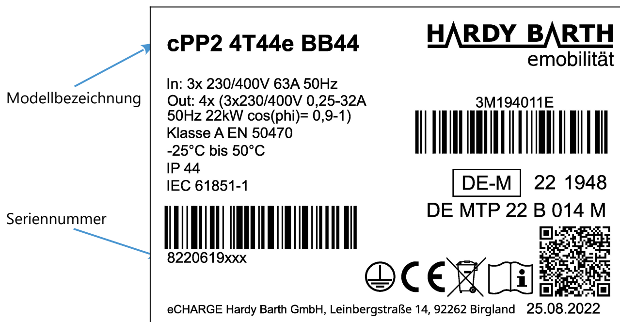
Abbildung 1: Typenschild cPP2
