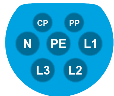
Abbildung 2: Typ 2 Stecker weiblich
