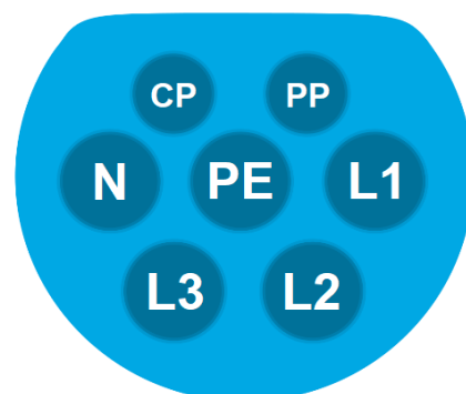
Abbildung 2: TYP 2 Stecker Weiblich
